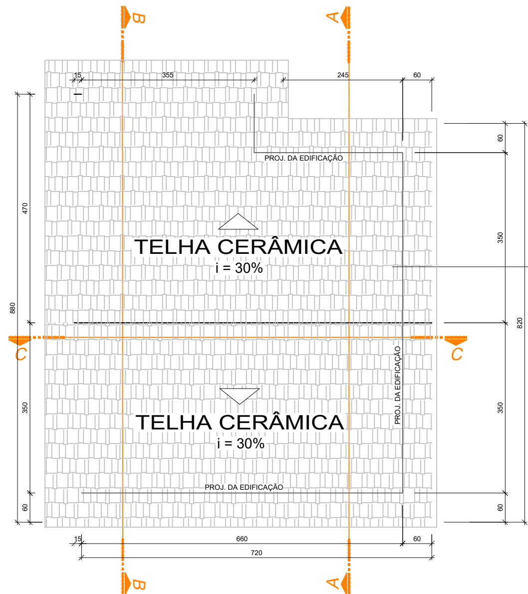
PLANTA DE COBERTURA - TIPO 05 ÁREA: 62,76m² (projeção da cobertura)
