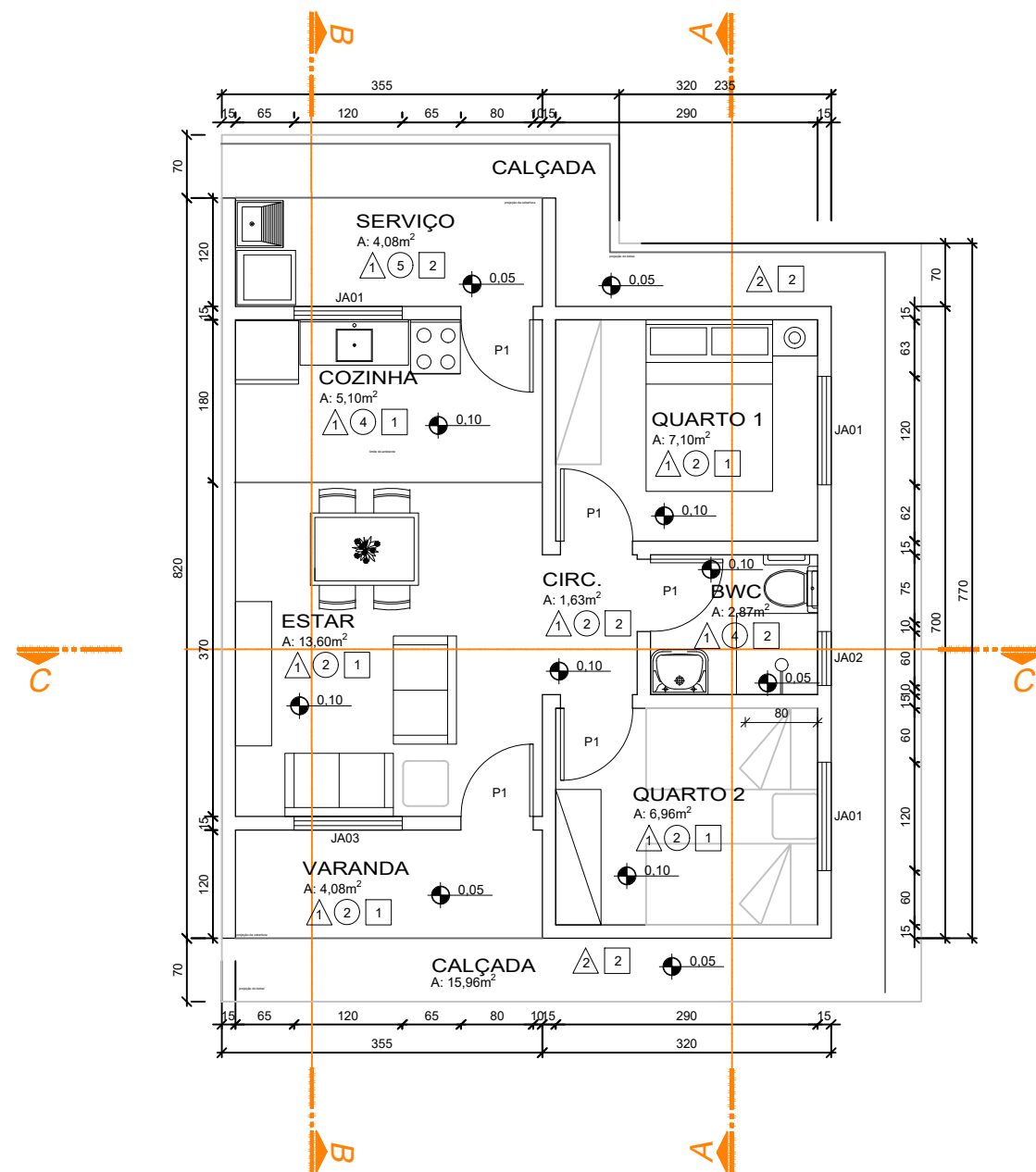
PLANTA BAIXA - TIPO 05 ÁREA: 42,99m² (51,69m² com varanda e serviço)
