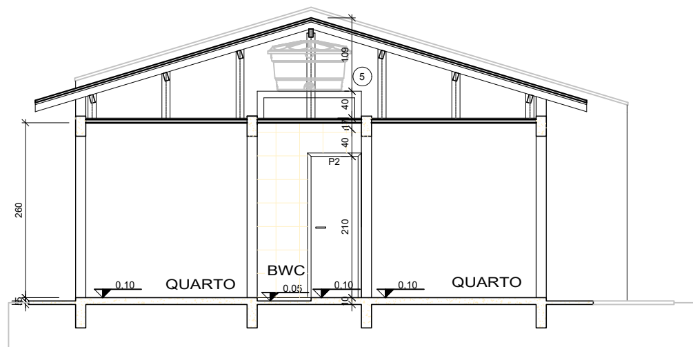
CORTE AA - TIPO 05
