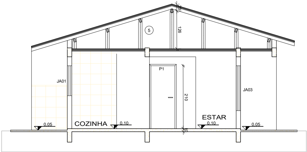
CORTE BB - TIPO 05
