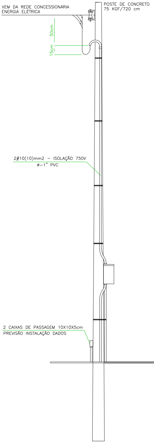
VISTA LATERAL
